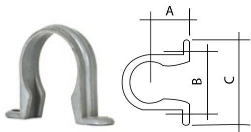
Pipe Clip
